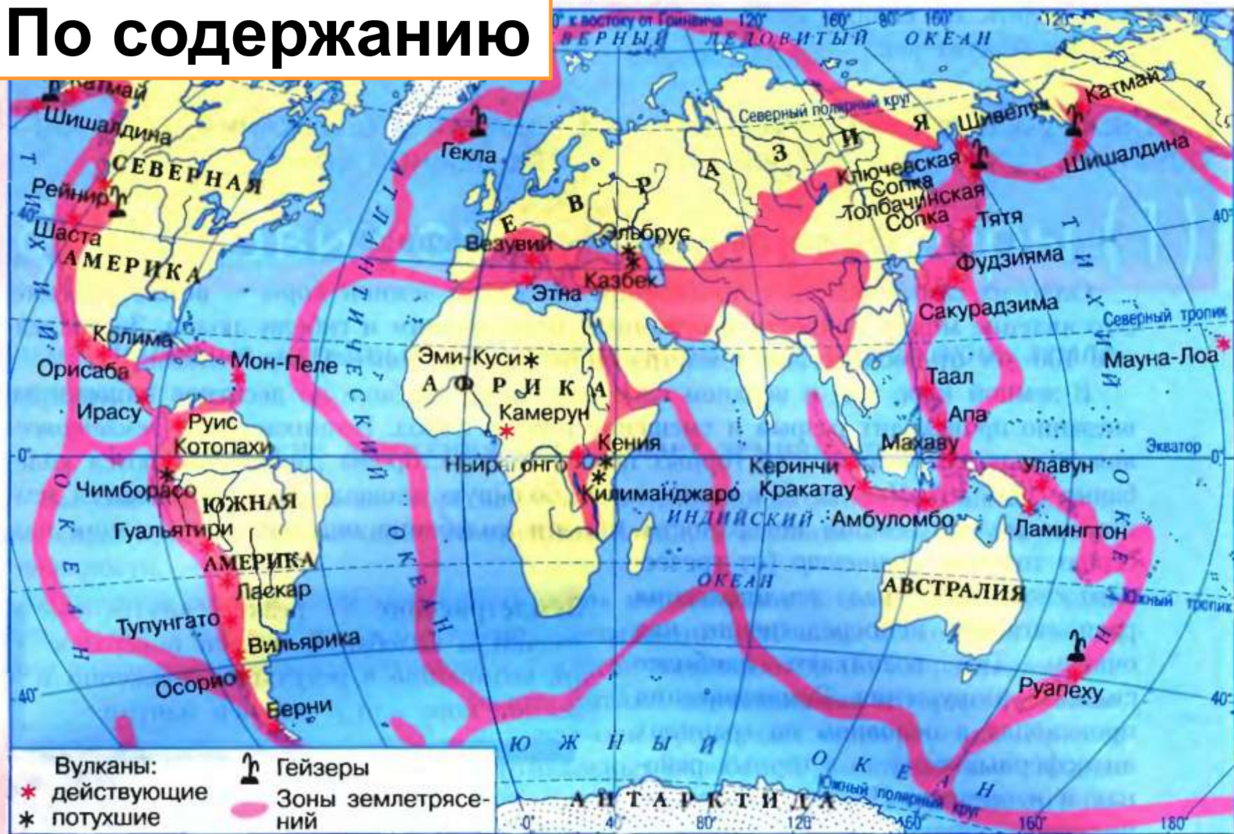
Рис. 50. Землетрясения и вулканизм
